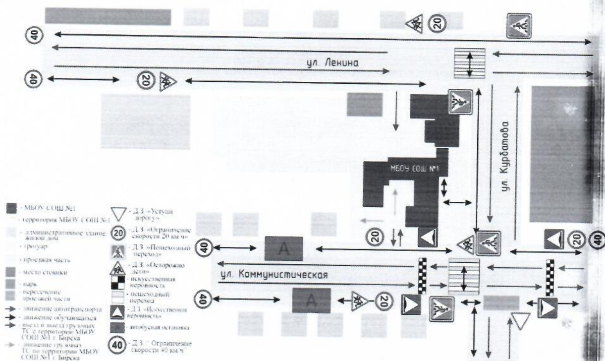
Схема организации дорожного движения в непосредственной близости от образовательного учреждения с размещением соответствующих технических средств организации дорожного движения, маршрутов движения детей и расположения парковочных мест.
